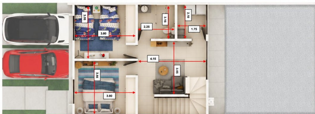
PLANTA ALTA
